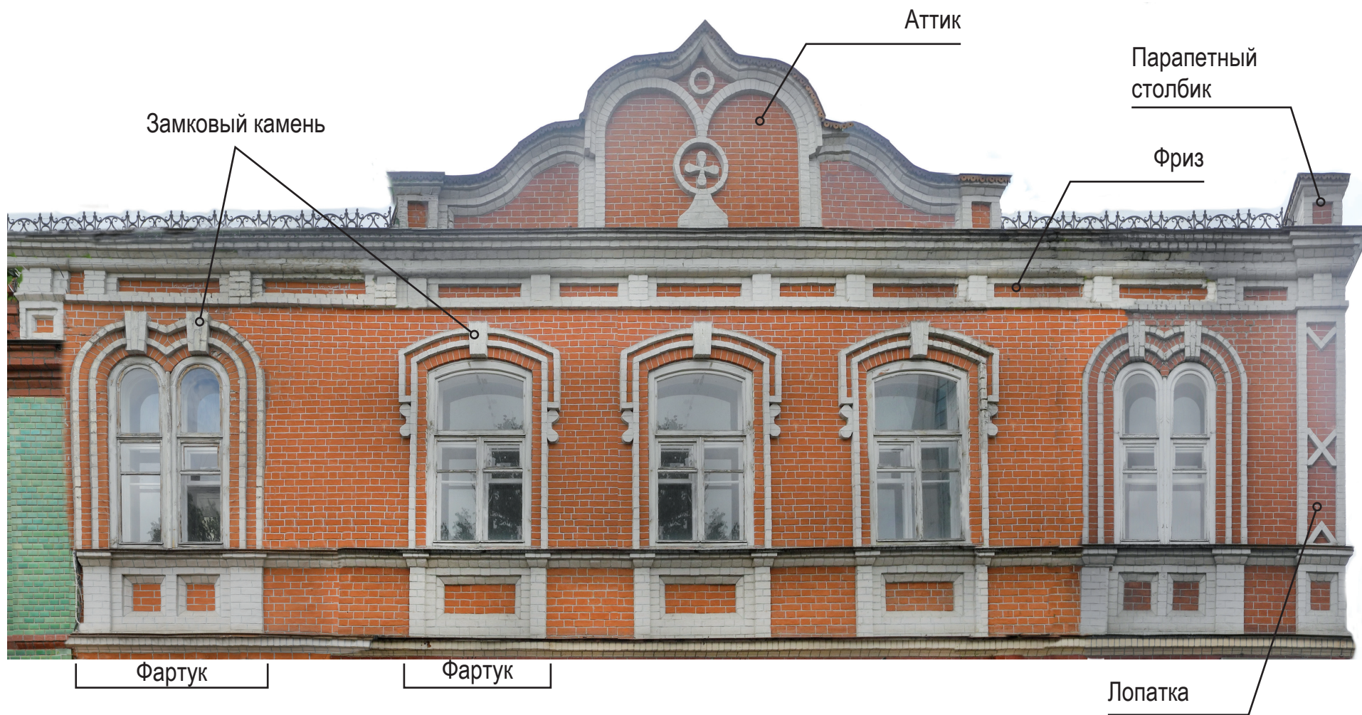
Фрагмент восточного фасада
